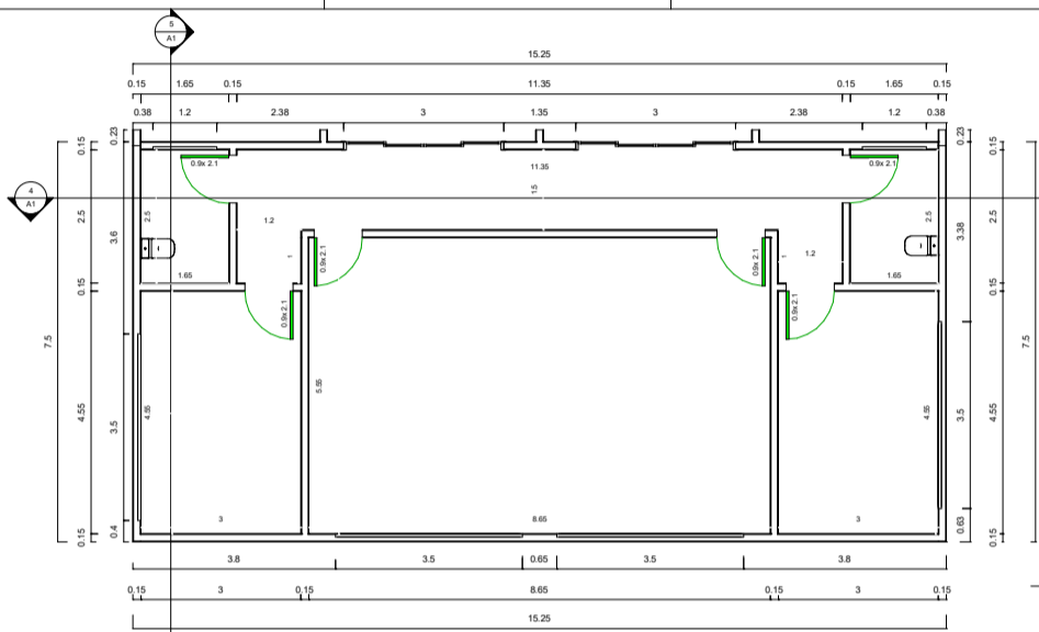
1 Planta Baixa 1 : 50
